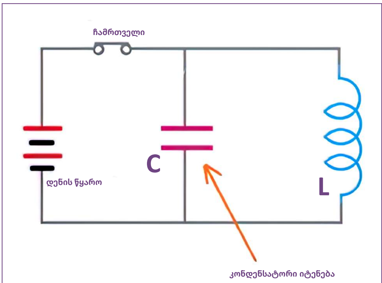
სურათი 86. რხევითი კონტური.
